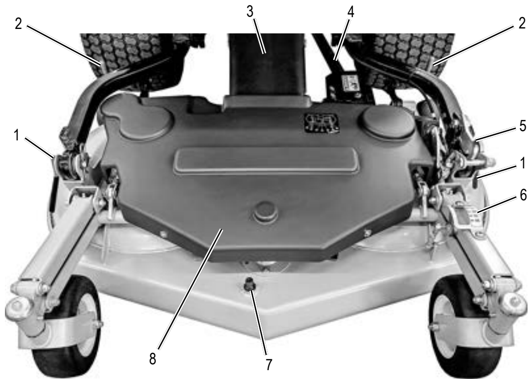
GETRIEBE SICHTBAR
