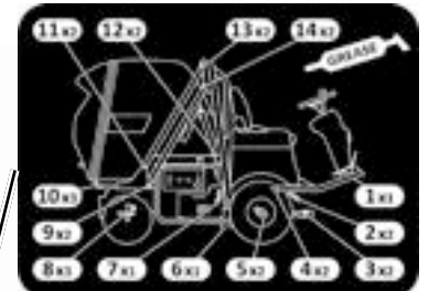
Maschinen Schmiernippel - Schema
